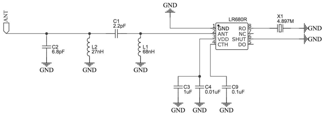
433.92 MHz 典型应用电路
