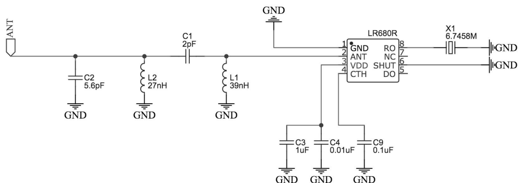
315 MHz 典型应用电路
