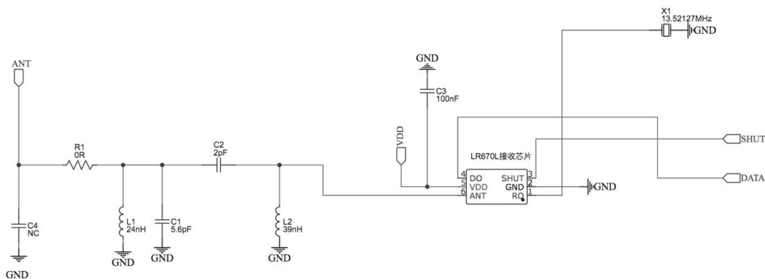
315 MHz 典型应用电路
