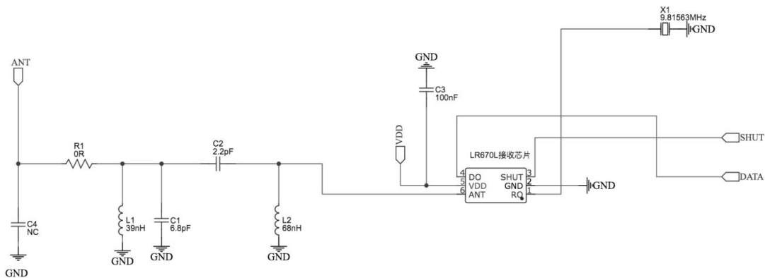
433.92 MHz 典型应用电路
